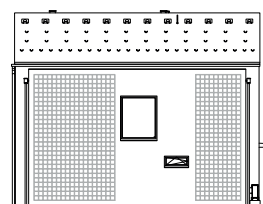
pohled jižní southern view
